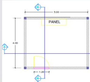
DENAH RUMAH PANEL
