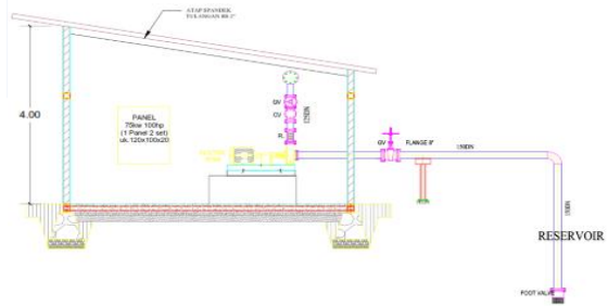
TAMPAK DEPAN Skala 1:50
